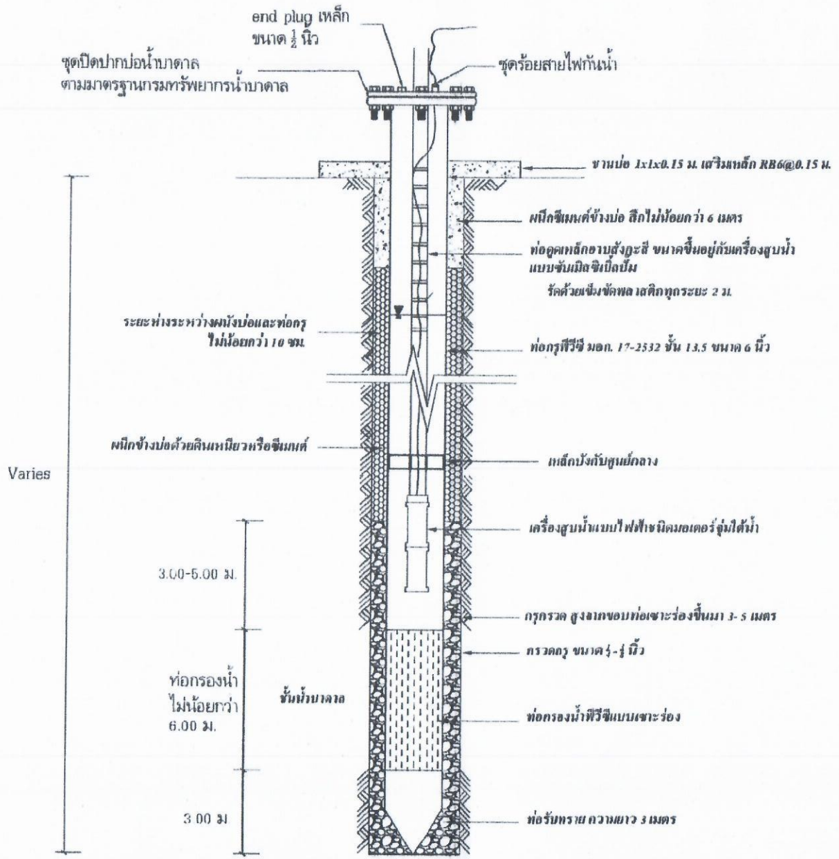
ภาพตัดบ่อน้ำบาดาล
